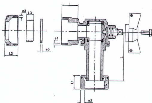
Hình ảnh minh họa 1 loại van góc liên hợp
