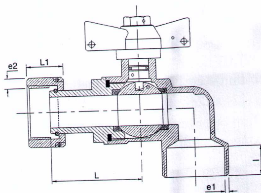
Hình ảnh minh họa 1 loại van góc
